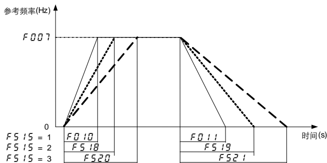
图 6.31 加/减速时间参数
