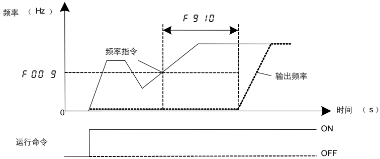
图 6.39 休眠唤醒示意图
