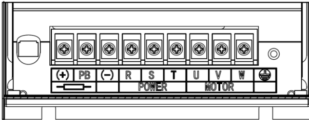
(b) 主回路功率端子 (15-22kW)
