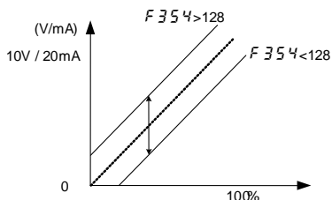
图 6.20 模拟输出曲线与 F354 关系
