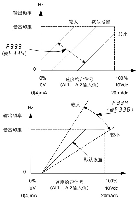
图 6.12 模拟输入校准
