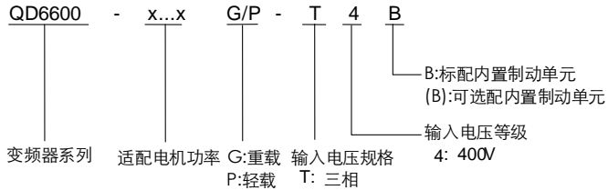
图 3.1 变频器型号说明示意图
