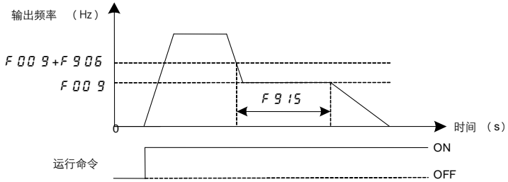
图 5.40 休眠模式进入
