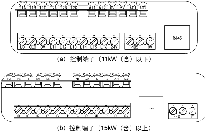
图 4.7 控制端子结构示意图
