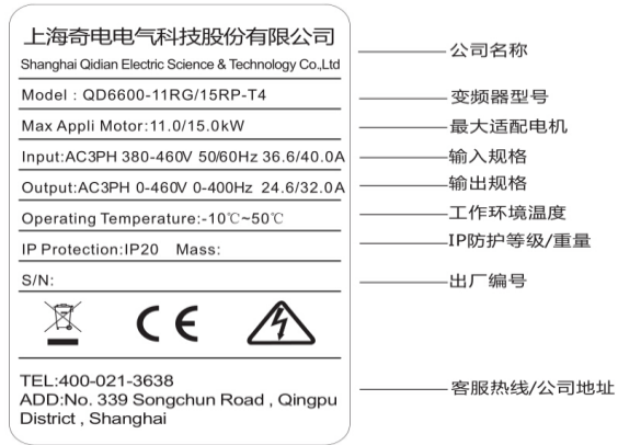
图 3.2 铭牌示例
