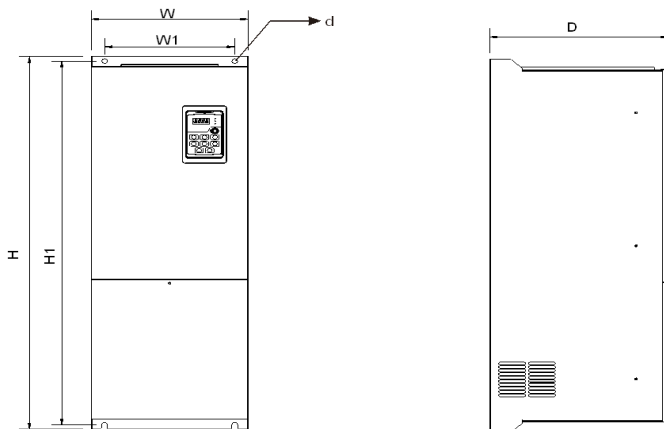
图 3.5 外形及安装尺寸示意图（三相 55KW-500KW）
