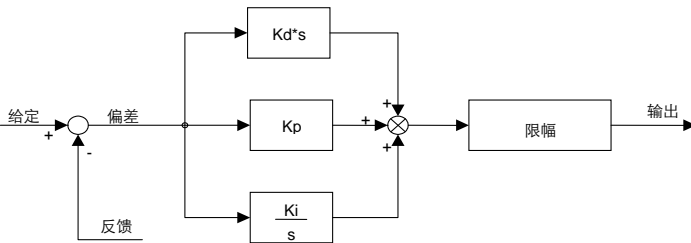
图 6.37 PID 调节器框图
