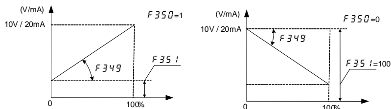
图 6.18 参数 F349 、 F350 和 F351 设置示意图
