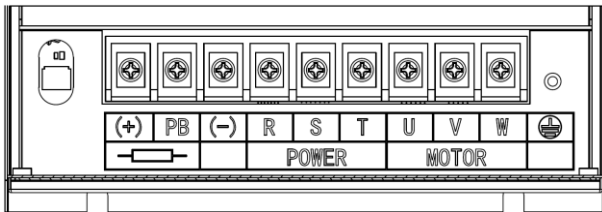
(c) 主回路功率端子 (30-37kW)
