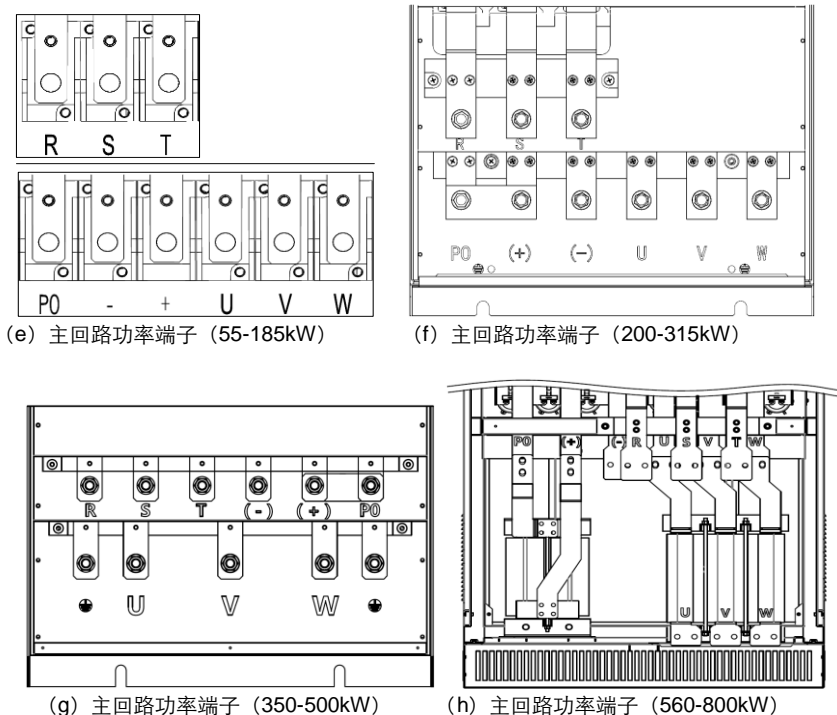
图 4.6 380V 产品主回路功率端子结构示意图
