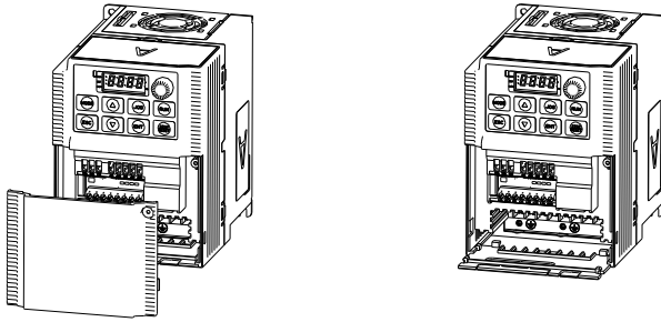
图 4.4 盖板、出线板的拆卸示意图
