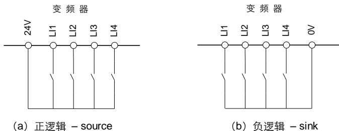
图 4.9 逻辑输入端子接线图
