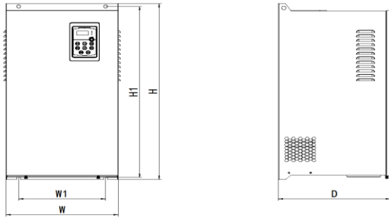
图 3.4 外形及安装尺寸示意图（三相 15KW-45KW）
