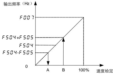
图 6.26 运行起始频率
