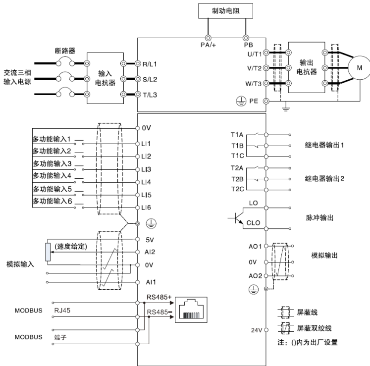
(a) 11kW (含) 以下标准接线图
