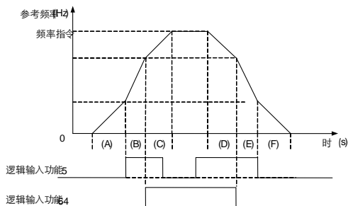
图 6.32 通过逻辑输入切换加减速曲线
